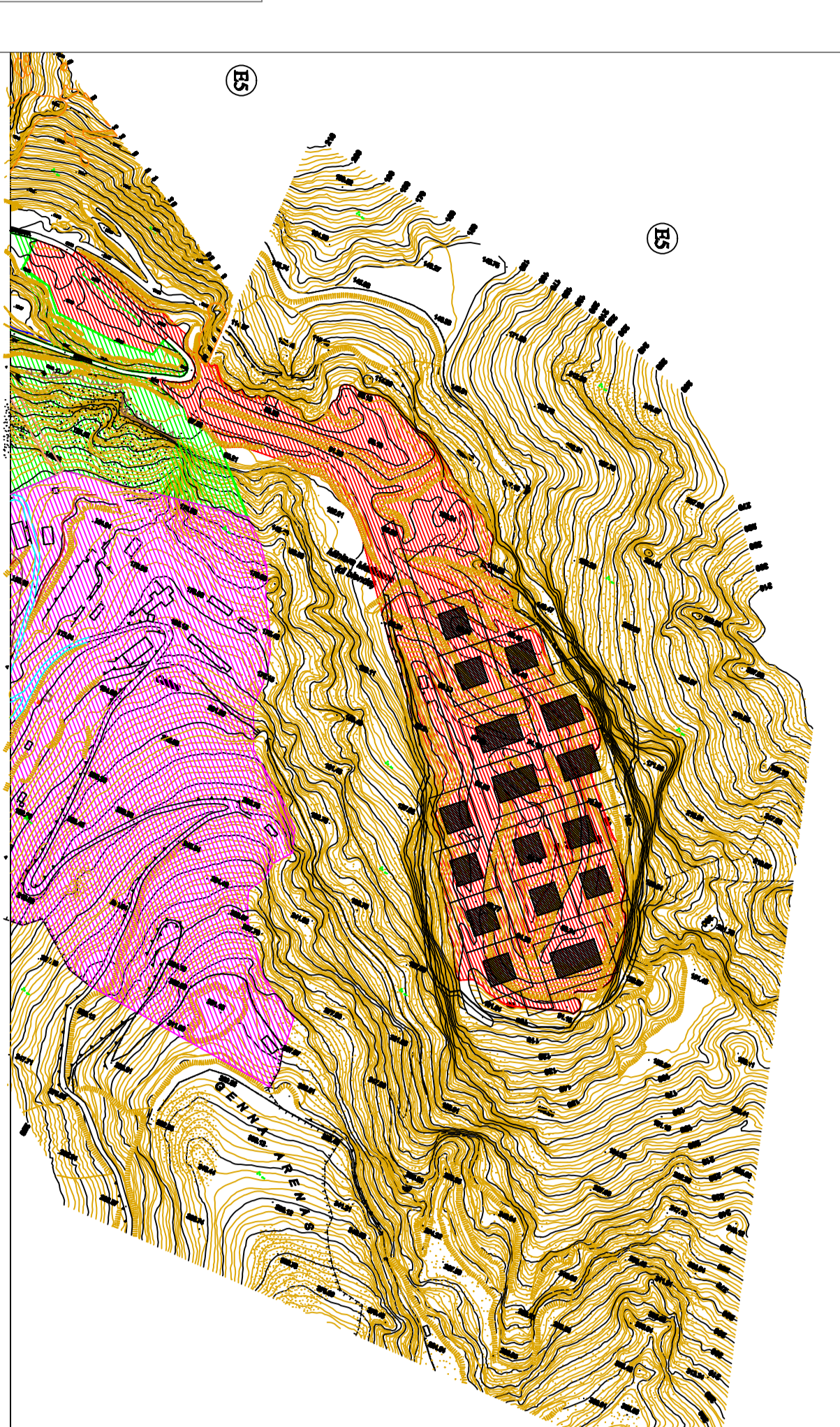
PLANIMETRIA STATO ATTUALE SC. 1:4000
